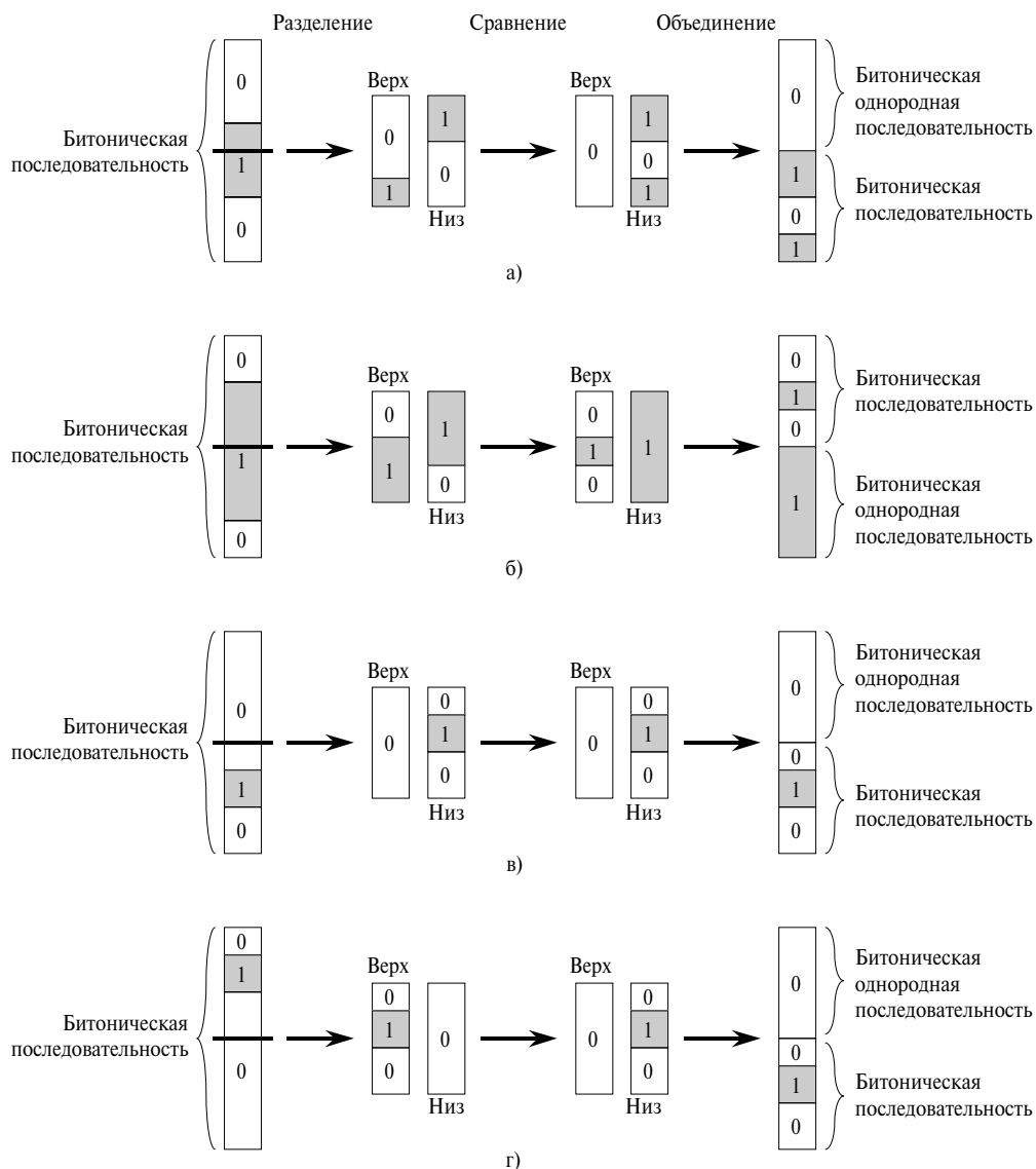
Рис. 27.8. Возможные частные случаи сравнения в сети HALF_CLEANER[n]
