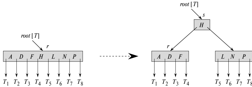
Рис. 18.6. Разбиение корня с t = 4
