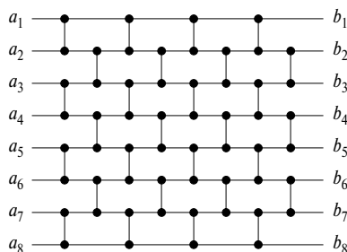
Рис. 27.13. Нечетно-четная сортирующая сеть на 8 входов
