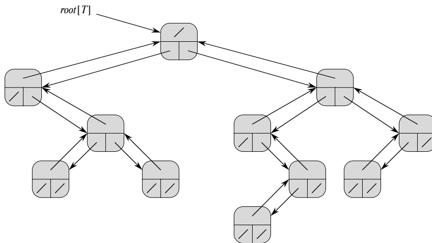
Рис. 10.9. Представление бинарного дерева T (поле key не показано)
