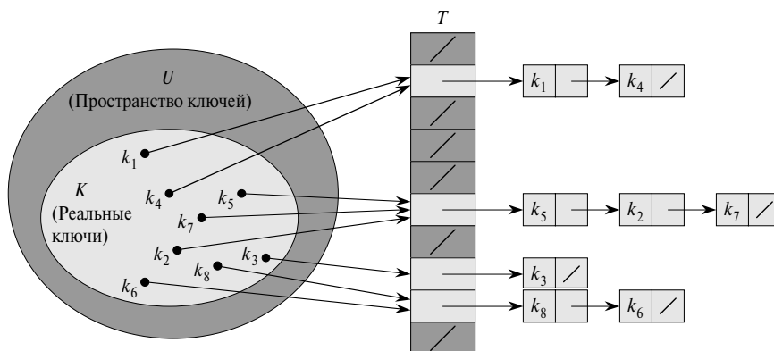
Рис. 11.3. Разрешение коллизий при помощи цепочек
