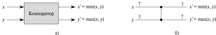
Рис. 27.1. Схематические представления сравнивающего устройства
