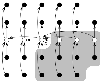
Рис. 9.1. Анализ алгоритма SELECT
