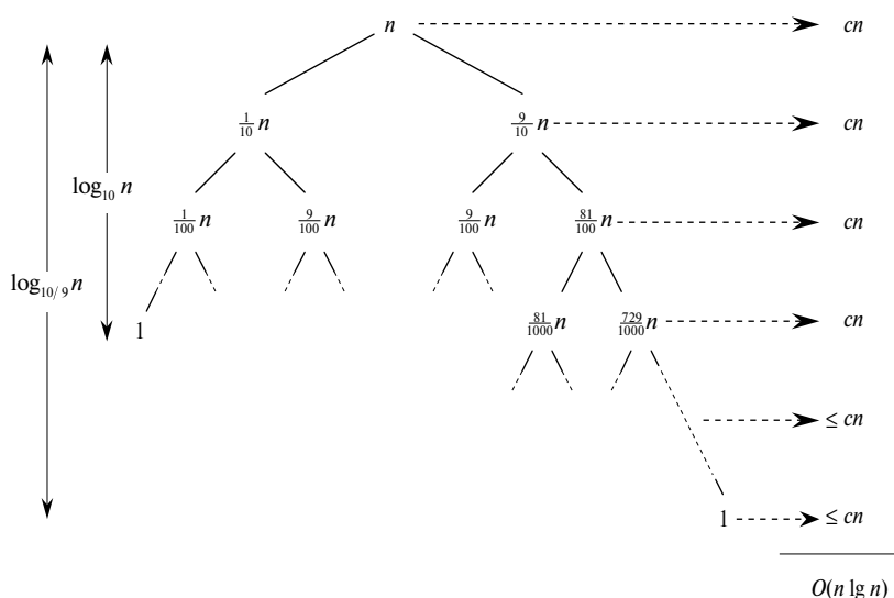
Рис. 7.4. Рекursive дерево, соответствующее делению задачи процедурой PARTITION в соотношении 1:9
