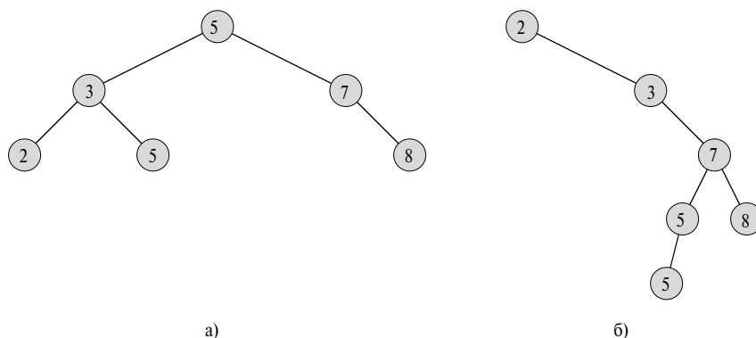
Рис. 12.1. Бинарные деревья поиска
