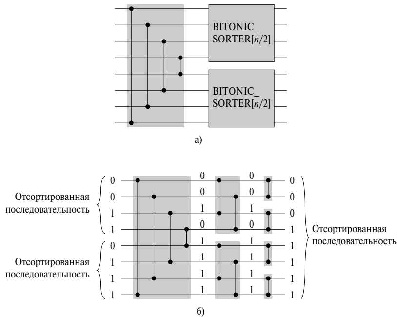
Рис. 27.11. Сеть, объединяющая две входные отсортированные последовательности, в одну выходную отсортированную последовательность при n = 8
