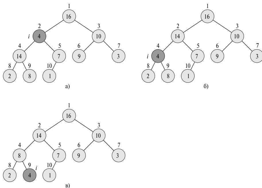
Рис. 6.2. Работа процедуры \text{MAX\_HEAPIFY}(A, 2) при \text{heap\_size}[A] = 10
