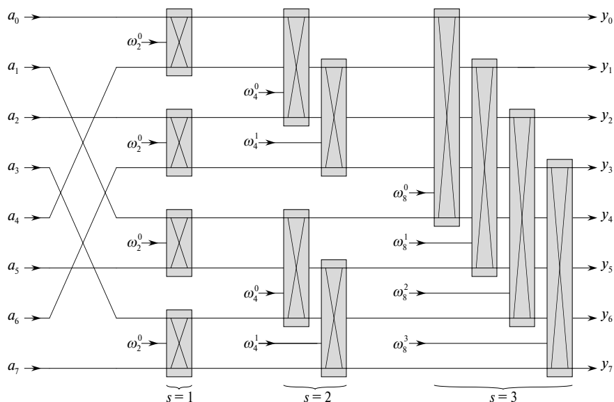
Рис. 30.5. Схема процедуры PARALLEL_FFT, вычисляющей БПФ при n = 8 .
