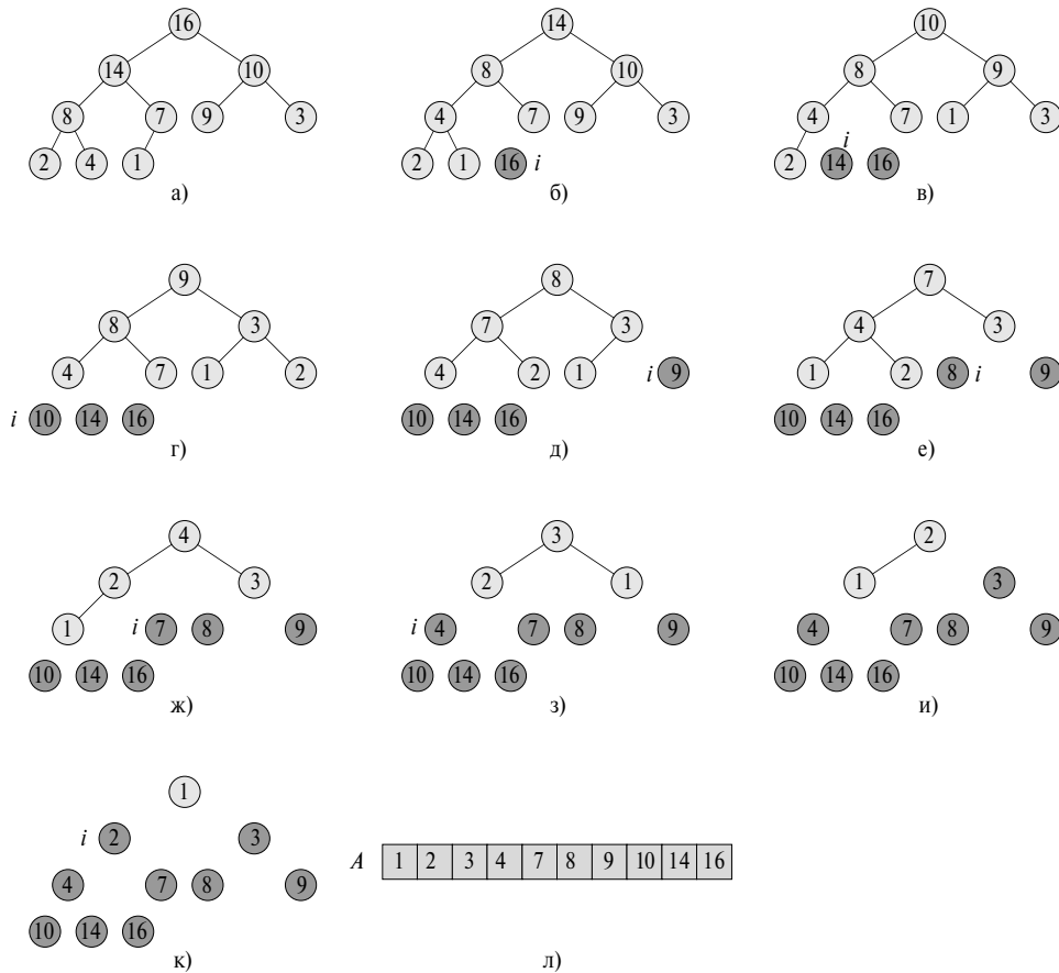
Рис. 6.4. Работа процедуры HEAPSORT
