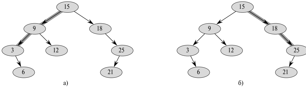
Рис. 13.11. Хребты в бинарных деревьях поиска (а — левый хребет, б — правый)
