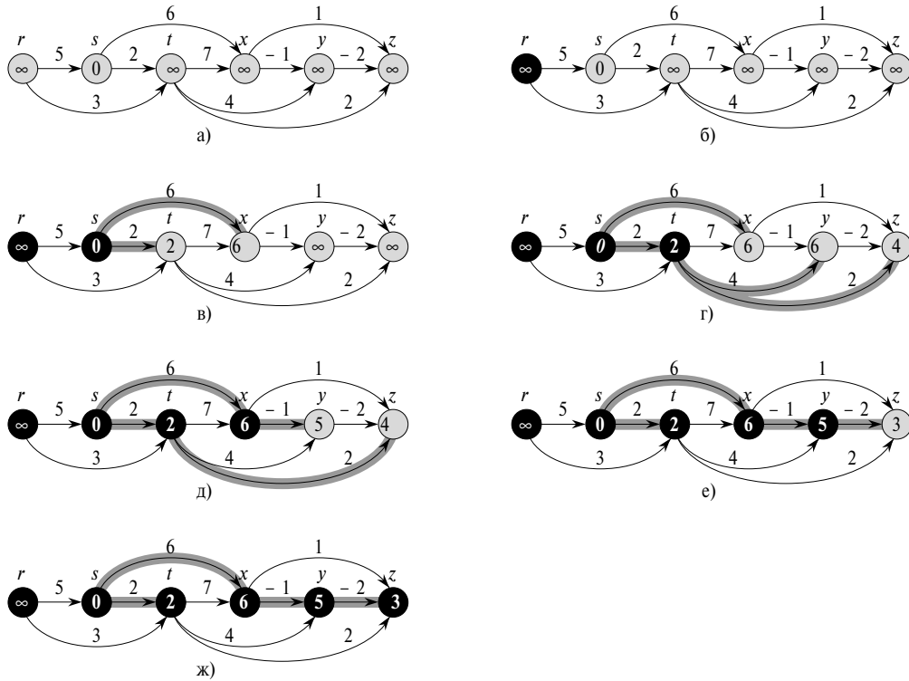
Рис. 24.5. Иллюстрация работы алгоритма, предназначенного для поиска кратчайших путей в ориентированном ациклическом графе
