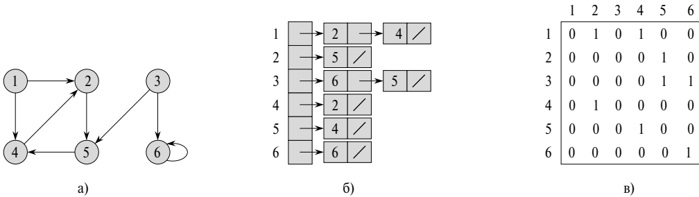
Рис. 22.2. Два представления ориентированного графа
