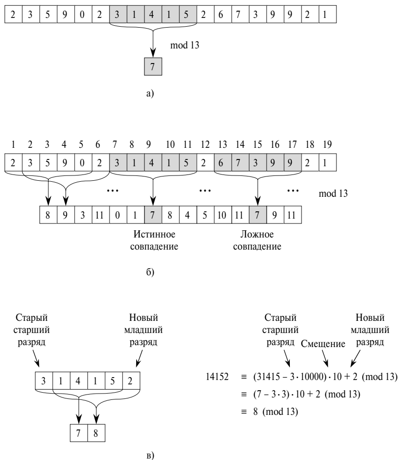
Рис. 32.4. Алгоритм Рабина-Карпа
