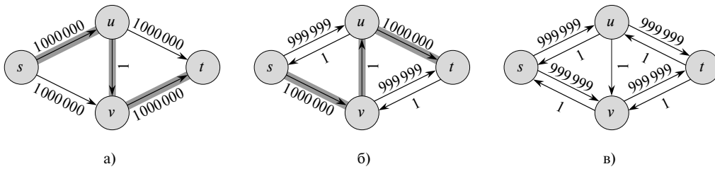
Рис. 26.6. Транспортная сеть, для которой выполнение процедуры FORD_FULKERSON может занимать время \Theta(E|f^*|) , |f^*| = 2\,000\,000
