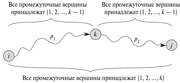
Рис. 25.3. Схема, иллюстрирующая структуру кратчайших путей
