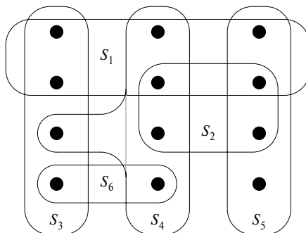
Рис. 35.3. Экземпляр (X, \mathcal{F}) задачи о покрытии множества, в котором множество X состоит из 12 черных точек, а \mathcal{F} = \{S_1, S_2, S_3, S_4, S_5, S_6\}
