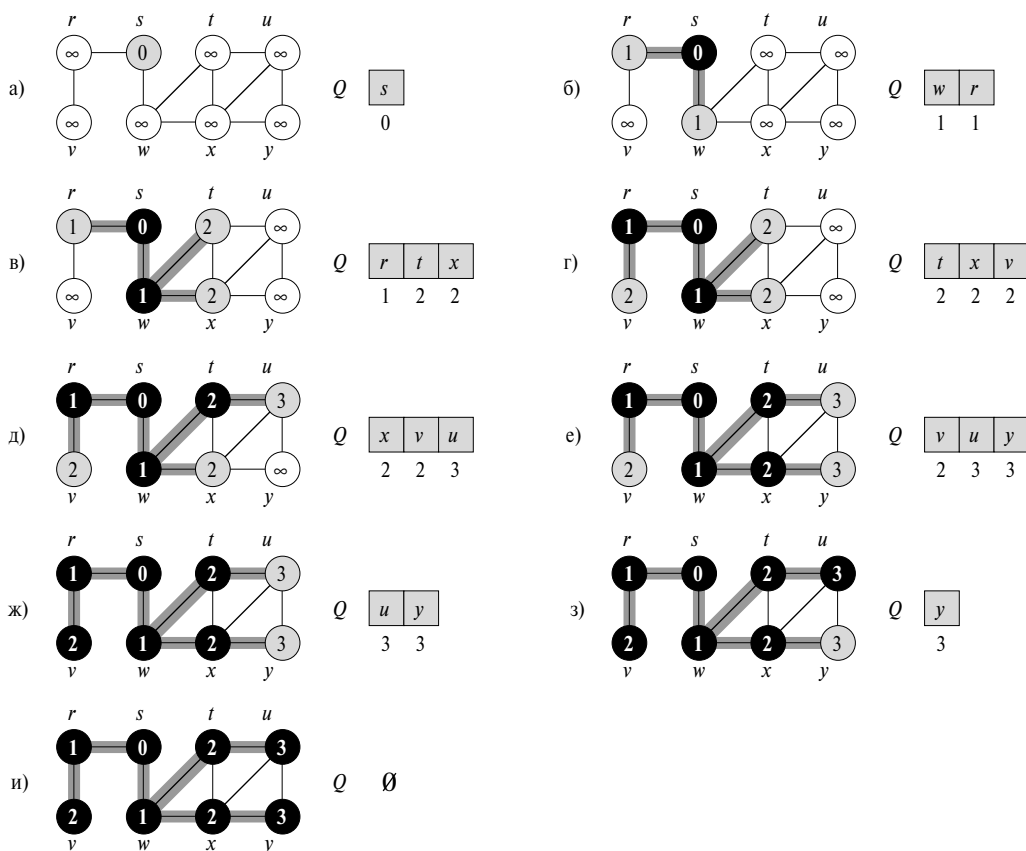
Рис. 22.3. Выполнение процедуры BFS над неориентированным графом
