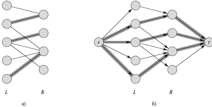
Рис. 26.8. Двудольный граф (а) и соответствующая ему транспортная сеть (б). Выделенные ребра обеспечивают максимальный поток и определяют максимальное паросочетание
