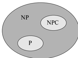
Рис. 34.6. Представление большинства специалистов в области вычислительных систем об отношении между классами P , NP и NPC ; классы P и NPC полностью содержатся в классе NP , и P \cap NPC = \emptyset
