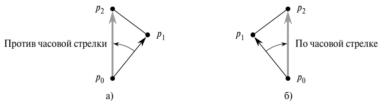
Рис. 33.2. Использование векторного произведения для определения направления поворота последовательных отрезков
