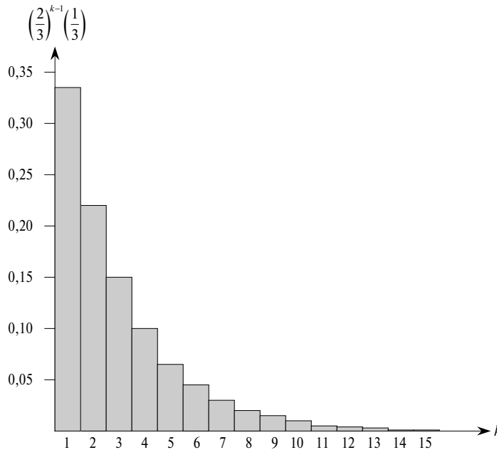
Рис. В.1. Геометрическое распределение с p = 1/3
