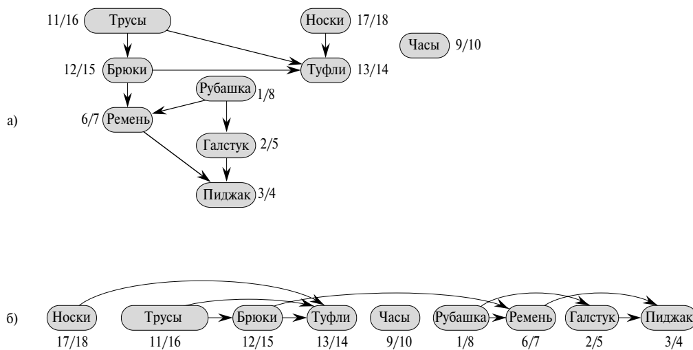
Рис. 22.7. Топологическая сортировка одежды
