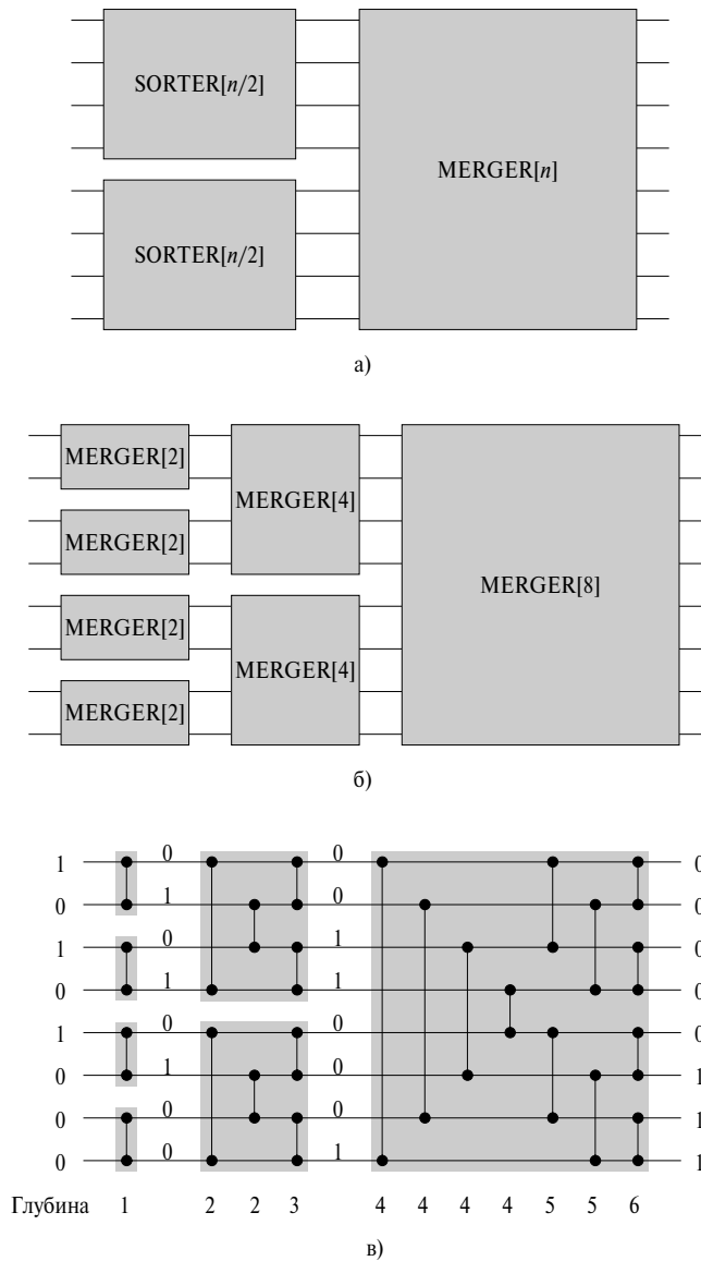
Рис. 27.12. Сортирующая сеть SORTER[n] , построенная путем рекурсивного совмещения объединяющих сетей
