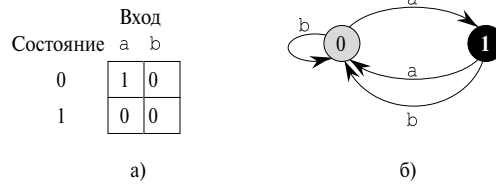
Рис. 32.5. Простой автомат с двумя состояниями: Q = \{0, 1\} , q_0 = 0 , \Sigma = \{a, b\}
