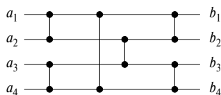
Рис. 27.6. Сортирующая сеть, предназначенная для сортировки четырех чисел
