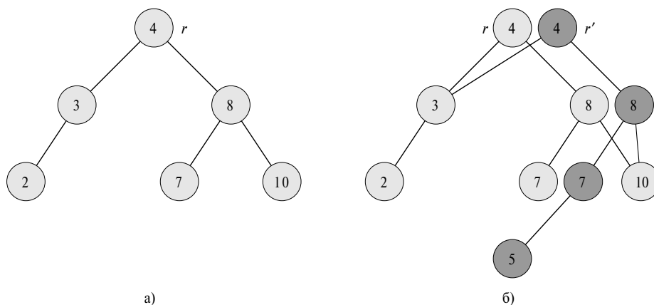
Рис. 13.8. Бинарное дерево поиска с ключами 2, 3, 4, 7, 8 и 10 (а) и перманентное бинарное дерево поиска, получающееся в процессе вставки ключа 5 (б)
