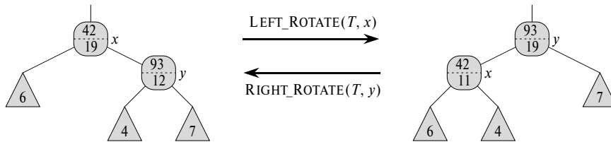
Рис. 14.2. Обновление размеров поддеревьев в процессе поворота
