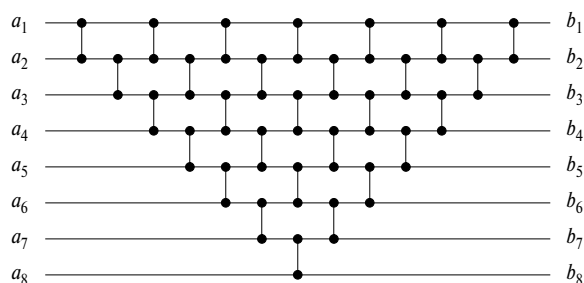
Рис. 27.3. Сортирующая сеть, основанная на методе сортировки вставками, для упражнения 27.1-6
