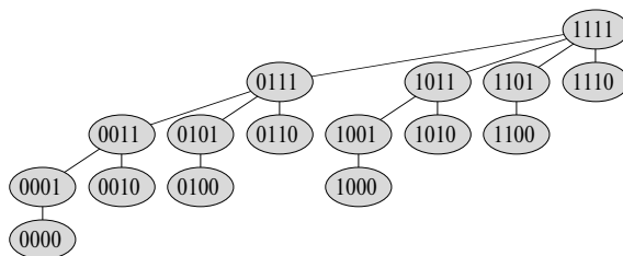
Рис. 19.3. Биномиальное дерево B_4 с узлами, помеченными двоичными числами при обходе в обратном порядке
