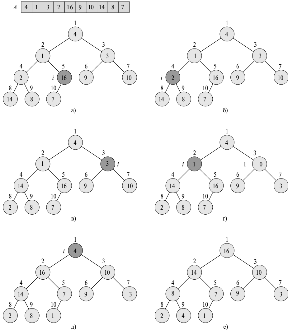
Рис. 6.3. Схема работы процедуры BUILD_MAX_HEAP
