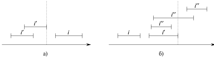
Рис. 14.5. Отрезки в доказательстве теоремы 14.2. Пунктирной линией показана величина \max[\text{left}[x]]
