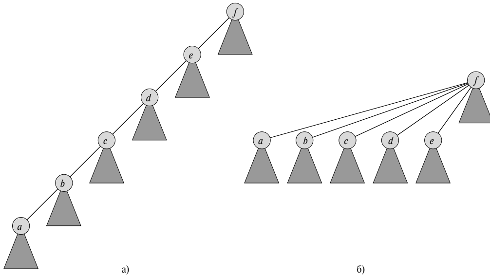
Рис. 21.4. Сжатие пути в процессе выполнения операции FIND_SET
