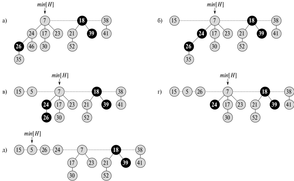
Рис. 20.4. Два вызова процедуры FIB_HEAP_DECREASE_KEY
