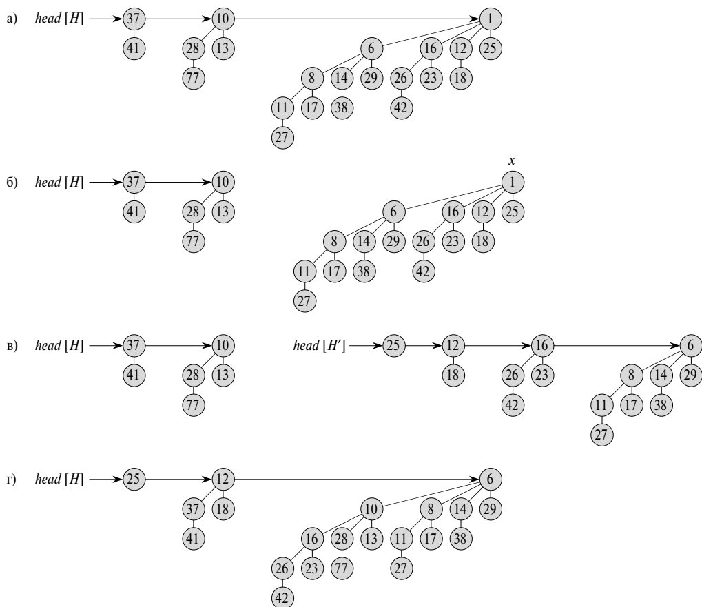
Рис. 19.6. Работа процедуры BINOMIAL_HEAP_EXTRACT_MIN
