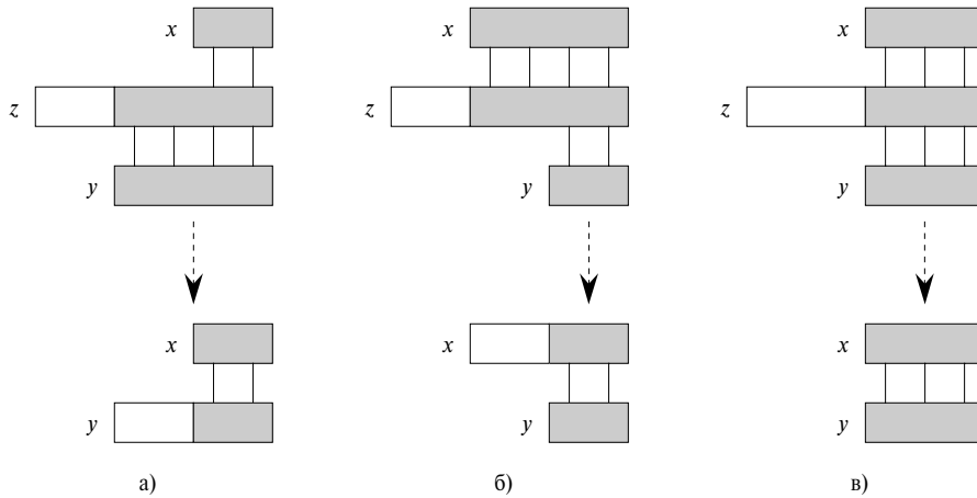
Рис. 32.2. Графическое доказательство леммы 32.1
