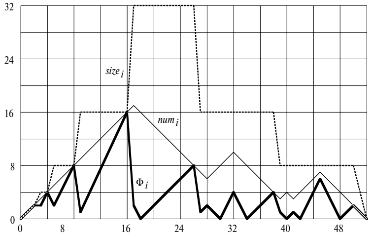
Рис. 17.4. Зависимость величин num_i (количество элементов в таблице), size_i (количество ячеек в таблице) и потенциала \Phi_i от количества операций TABLE_INSERT и TABLE_DELETE
