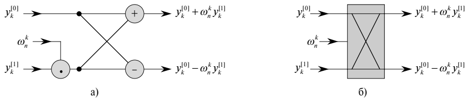
Рис. 30.3. Преобразование бабочки. а) Слева поступают два входимых значения, \omega_n^k умножается на y_k^{[1]} , соответствующие сумма и разность выводятся справа. б) Упрощенная схема преобразования бабочки, используемая в параллельной схеме БПФ
