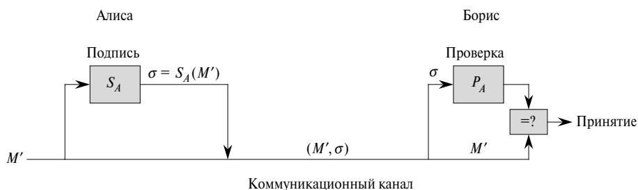
Рис. 31.2. Цифровые подписи в системе с открытым ключом
