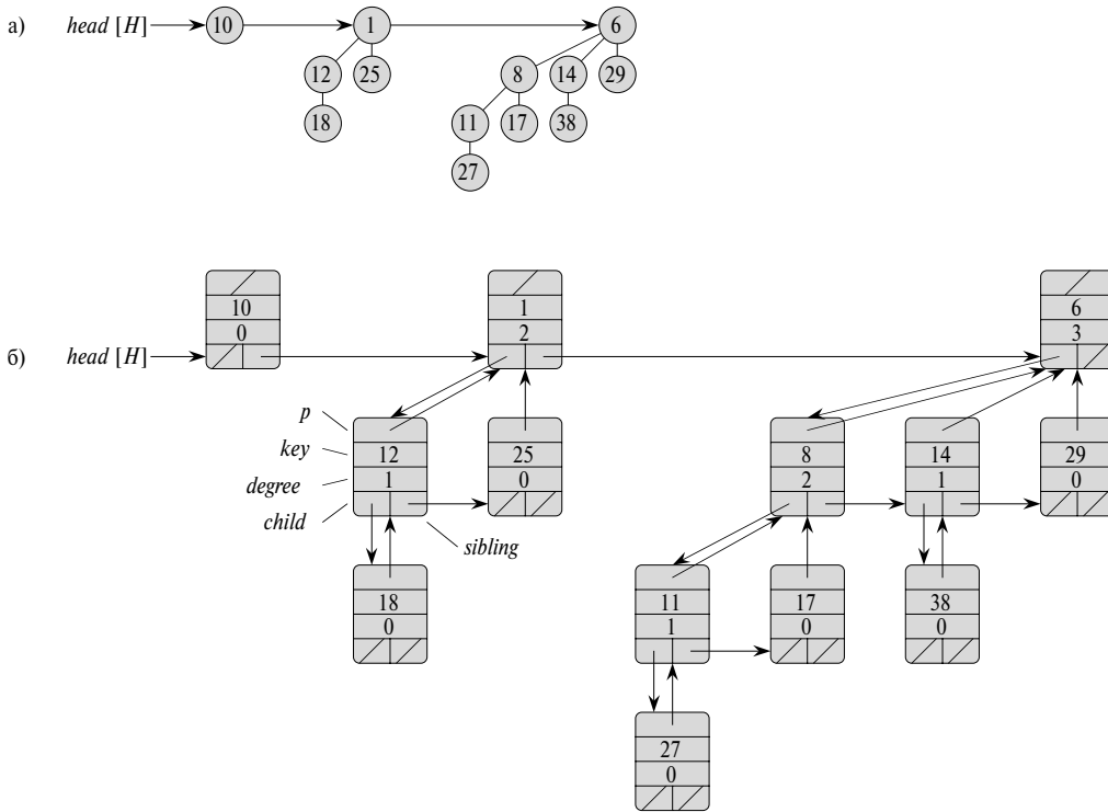
Рис. 19.2. Биномиальная пирамида с 13 узлами
