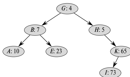
Рис. 13.9. Дерамида. Каждый узел имеет метку key[x] : priority[x]
