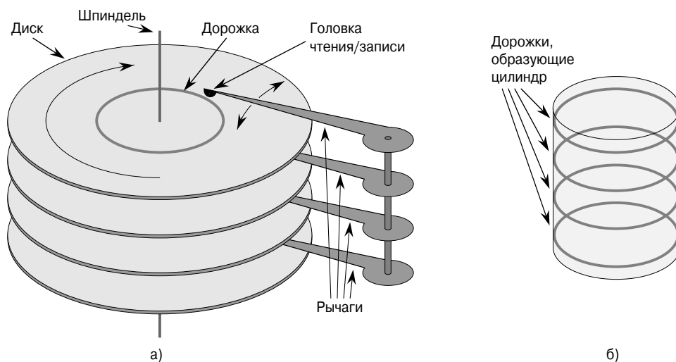
Рис. 18.2. Типичный дисковый накопитель
