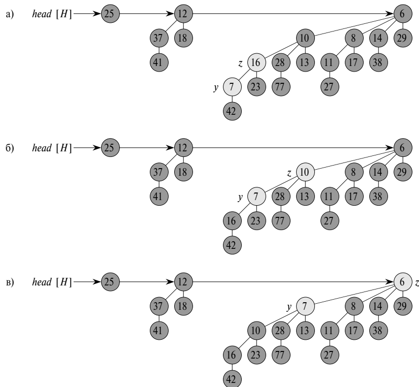
Рис. 19.7. Работа процедуры BINOMIAL_HEAP_DECREASE_KEY
