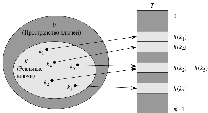
Рис. 11.2. Использование хеш-функции h для отображения ключей в ячейки хеш-таблицы. Ключи k_2 и k_5 отображаются в одну ячейку, вызывая коллизию
