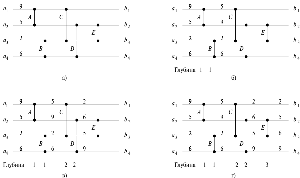
Рис. 27.2. Сравняющая сеть на 4 входа и 4 выхода, которая фактически является сортирующей сетью
