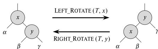
Рис. 13.2. Операции поворота в бинарном дереве поиска
