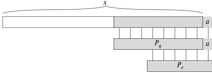
Рис. 32.8. Иллюстрация к доказательству леммы 32.3; из рисунка видно, что выполняется соотношение r = \sigma(P_q a) , где q = \sigma(x) и r = \sigma(xa)
