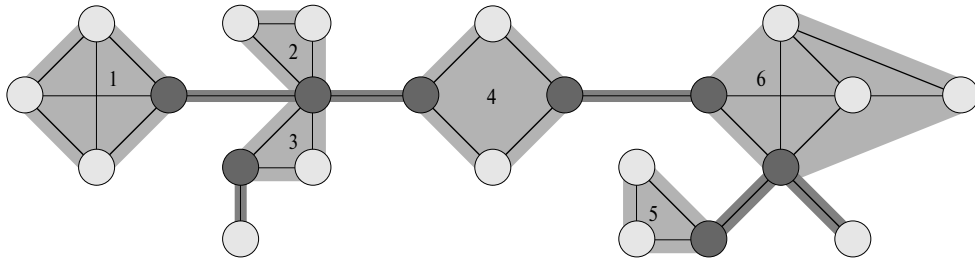
Рис. 22.10. Точки сочленения, мосты и двусвязные компоненты связного неориентированного графа
