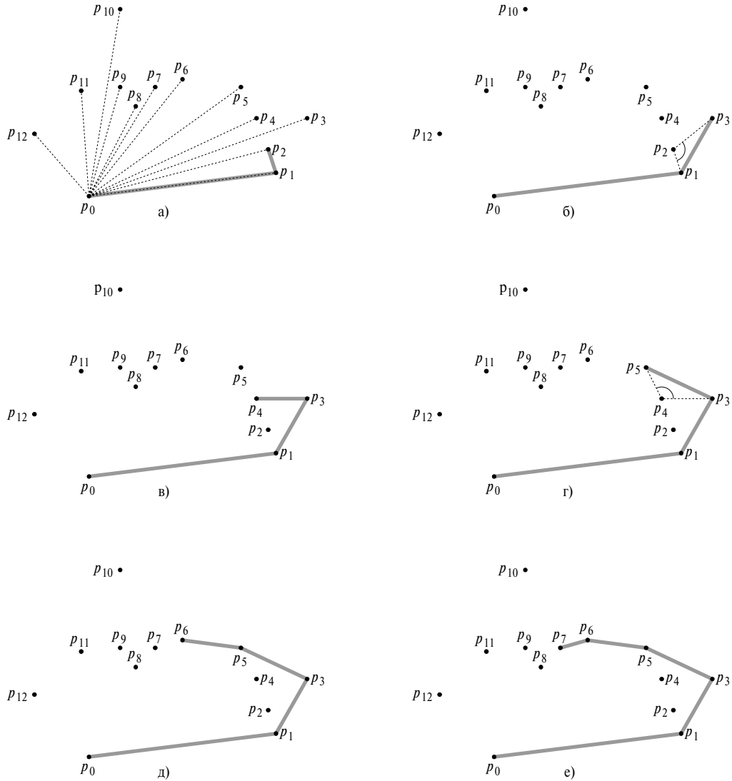
Рис. 33.7. Обработка процедурой GRAHAM_SCAN множества точек Q , показанного на рис. 33.6
