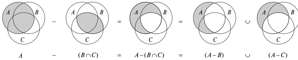
Рис. Б.1. Диаграмма Венна, иллюстрирующая первый закон де Моргана
