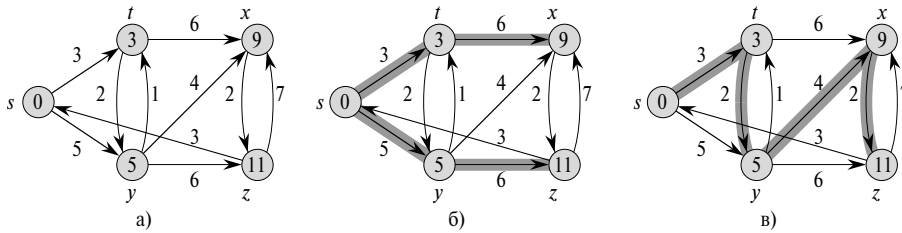
Рис. 24.2. Два разных дерева кратчайших путей, соответствующих одному и тому же взвешенному ориентированному графу
