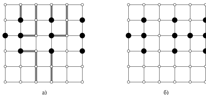
Рис. 26.11. Решетки для задачи о выходе. Стартовые точки отмечены черным цветом, остальные вершины решетки белые. а) Решетка с выходом, пути указаны цветом. б) Решетка без выхода
