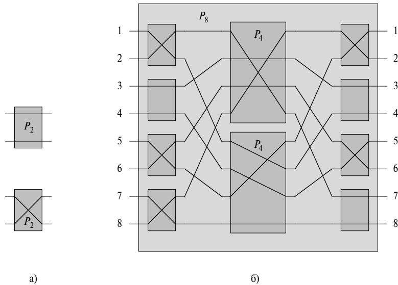
Рис. 27.14. Перестановочная сеть
