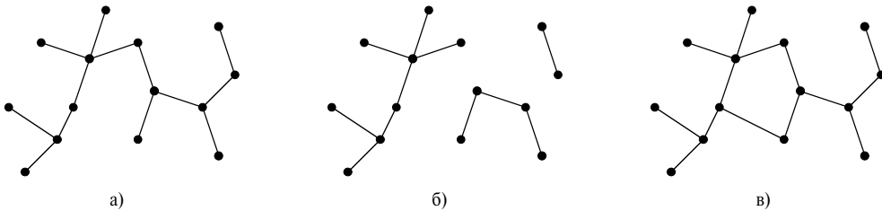
Рис. Б.4. Примеры дерева, леса и графа, который не является деревом или лесом из-за наличия цикла
