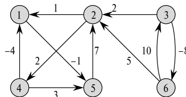
Рис. 25.2. Взвешенный ориентированный граф, который используется в упражнениях 25.1-1, 25.2-1 и 25.3-1
