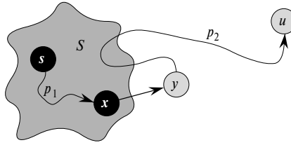
Рис. 24.7. Иллюстрация к доказательству теоремы 24.6
