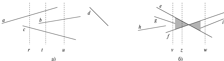
Рис. 33.4. Упорядочение отрезков с помощью разных вертикальных выметающих прямых
