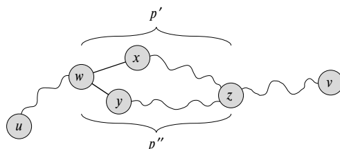
Рис. Б.5. Иллюстрация к доказательству теоремы Б.2
