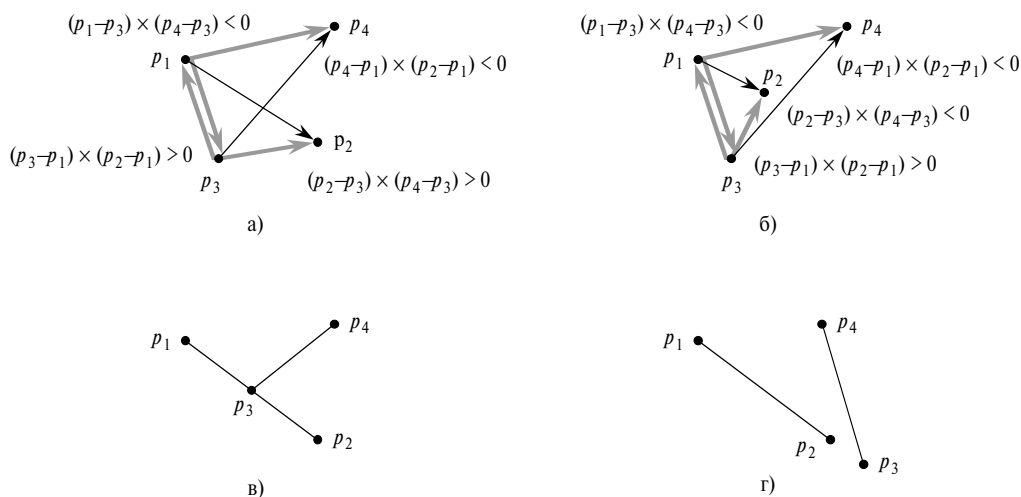
Рис. 33.3. Частные случаи в процедуре SEGMENTS_INTERSECT
