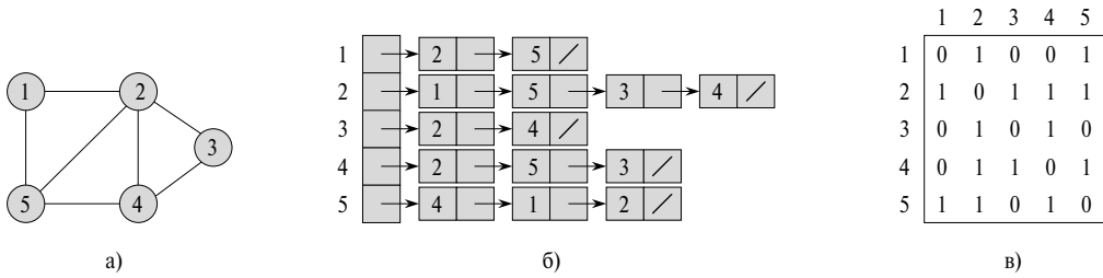
Рис. 22.1. Два представления неориентированного графа
