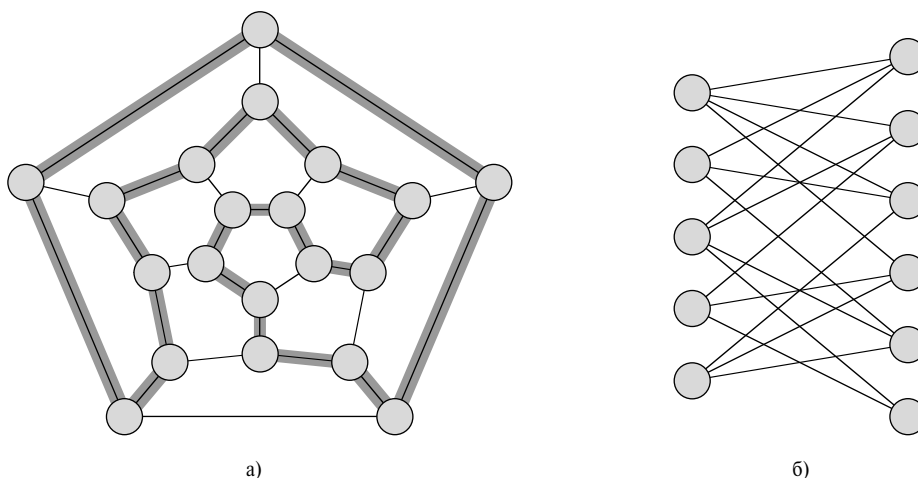
Рис. 34.2. Примеры гамильтонового (а) и негамильтонового (б) графов
