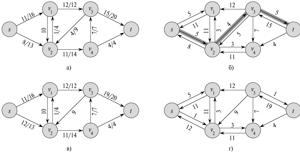
Рис. 26.3. а) Транспортная сеть G и поток f , представленные на рис. 26.1б. б) Остаточная сеть G_f с выделенным увеличивающим путем; его остаточная пропускная способность равна 4. в) Поток в сети G , полученный в результате увеличения потока вдоль пути p на величину его остаточной пропускной способности 4. г) Остаточная сеть, порожденная потоком, показанным в части в)
