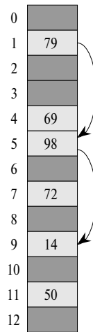
Рис. 11.5. Вставка при двойном хешировании
